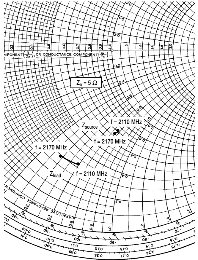
MRF6S21100NBR1
